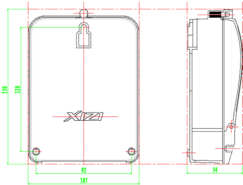
安装图
