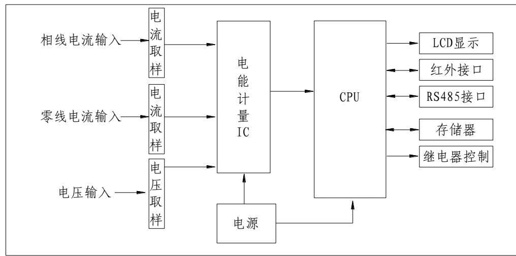
图1 DDZY601型单相费控智能电能表原理框图
