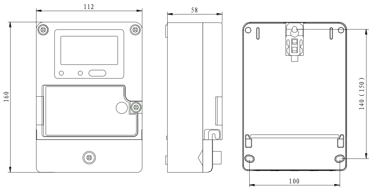
图4 DDZY601型单相费控智能电能表外形及安装尺寸图
