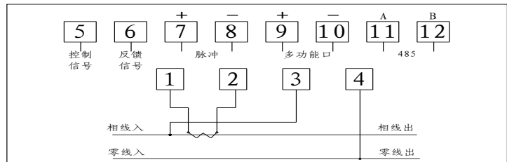
图3 DDZY601型单相费控智能电能表(互感式)接线图
