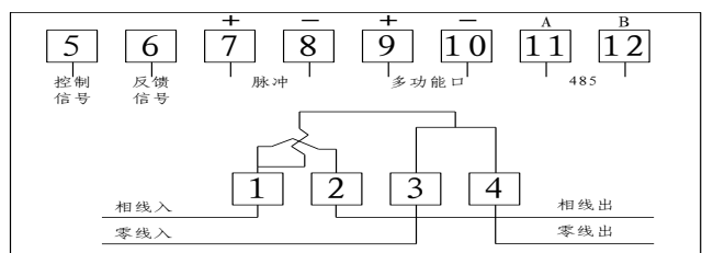
图2 DDZY601型单相费控智能电能表(直接式)接线图
